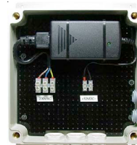
Art.Nr. 14359 mit 12V DC / 2,5A Netzteil
